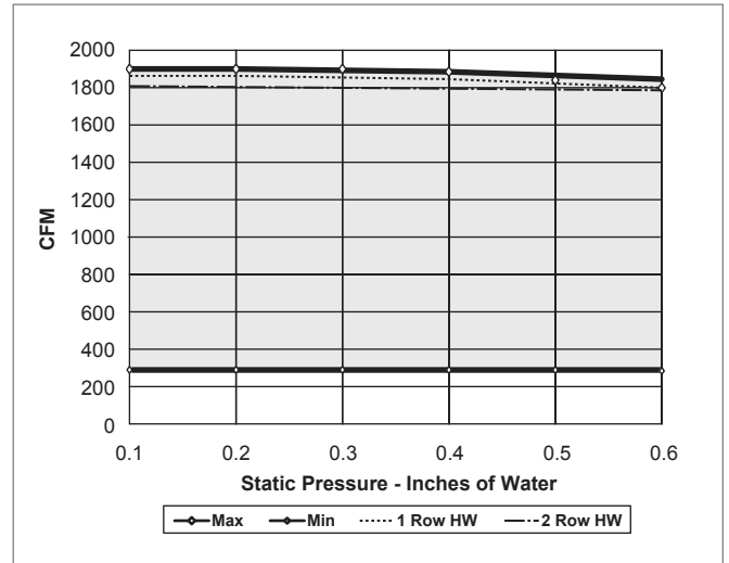
KLPS, ECM FAN CURVE, UNIT SIZE 4
