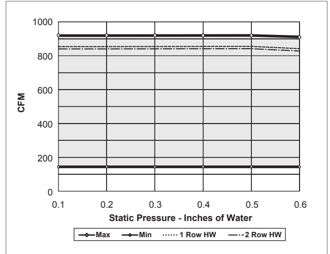
KLPS, ECM FAN CURVE, UNIT SIZE 2
