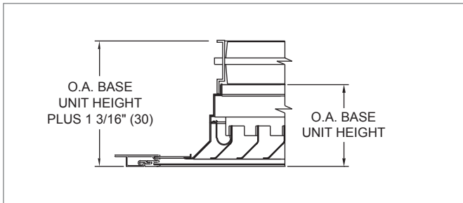
51240P, OBD DETAIL
