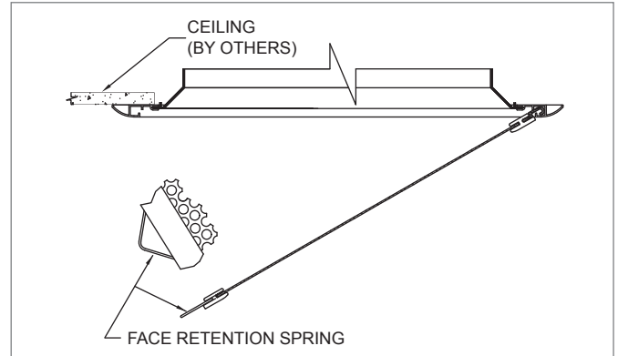
51240P, HINGE DETAIL
