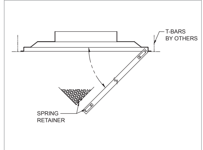
6600FR, HINGE DETAIL
