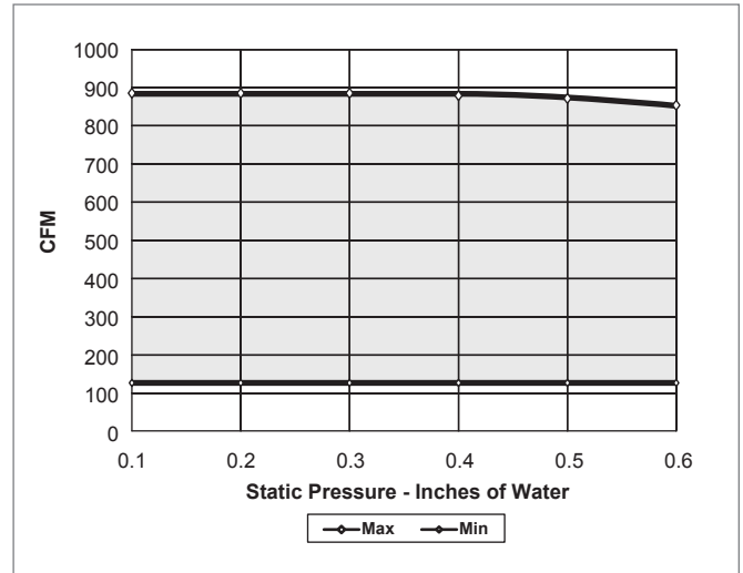
KLPP, ECM FAN CURVE, UNIT SIZE 4
