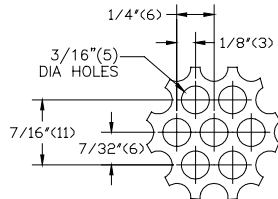
PERF DETAIL
