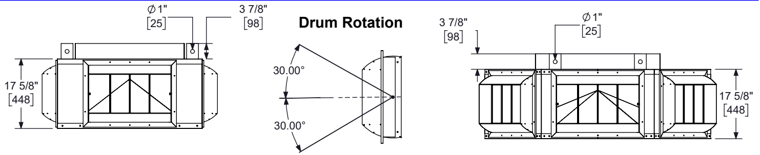
6 Outlet
