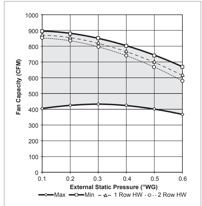
KLPP, PSC FAN CURVE, UNIT SIZE 4
